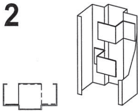
2 METAL STUD
